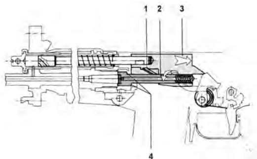
Figura 17: sbloccaggio dell'otturatore
