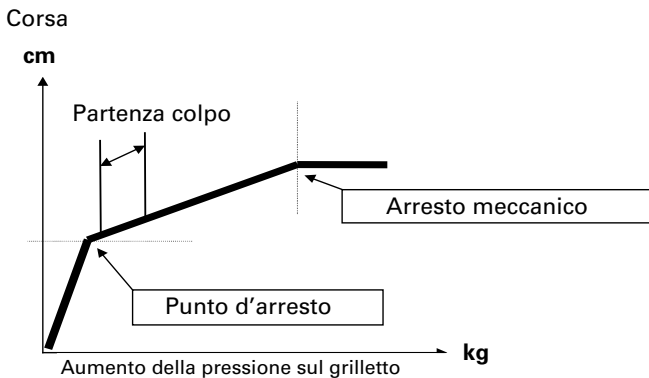
Figura 26: variazione della pressione sul grilletto in funzione della corsa
