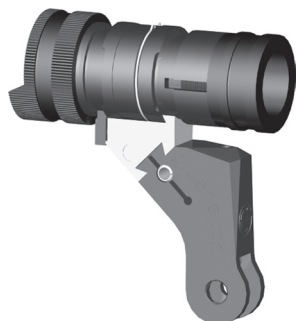
Bild 24: Universalkornträger zu Stgw 57 (Normalmontage), diverse Fabrikate
