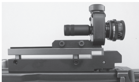
Bild 27: Diopferträger zu Stgw 57 zur Aufnahme schussfester Diopfer, diverse Fabrikate
